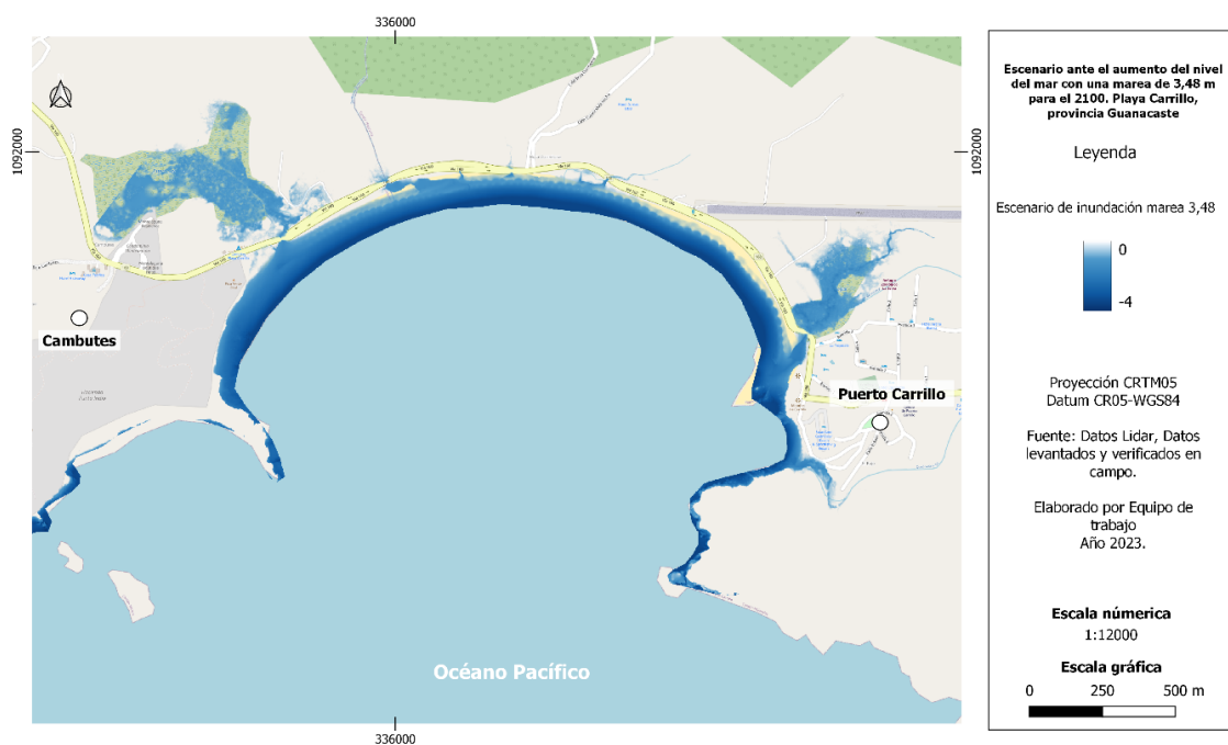
Figura 10. Escenarios de vulnerabilidad ante el aumento del nivel del mar. Marea 3.48 m
