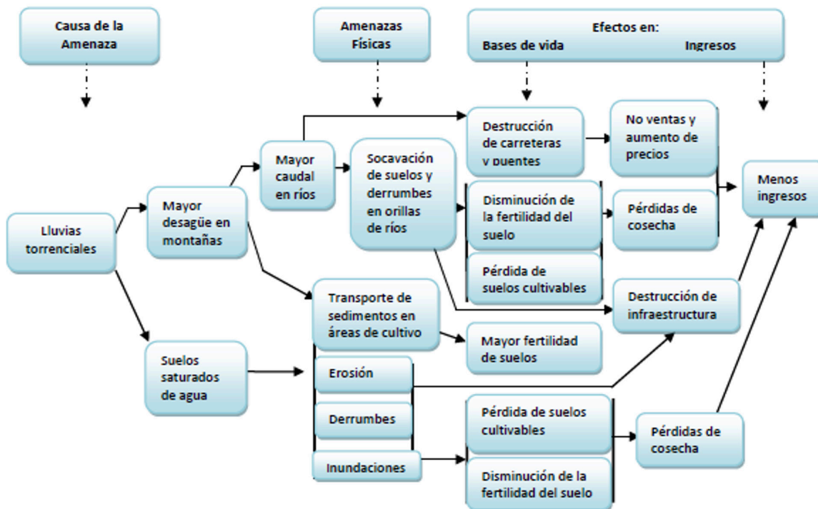
Figura 17. Cadena causa efecto de las lluvias torrenciales para la caficultura del cantón:
