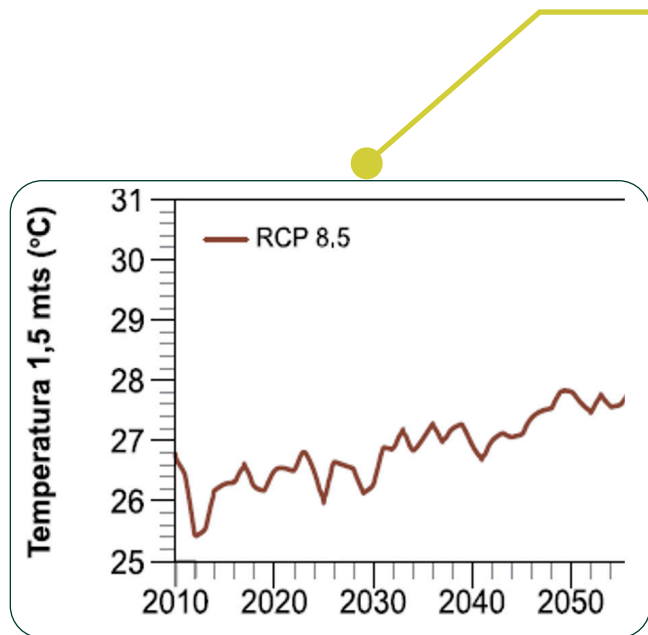
Figura 10. Proyección de la variación temporal de la temperatura para el período 2010-2050.
