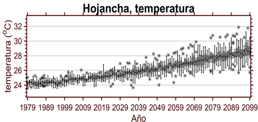
Figura 14. Valores anuales proyectados bajo un escenario pesimista de concentraciones en la temperatura de 1979 a 2099 promediado para todo el cantón 1
