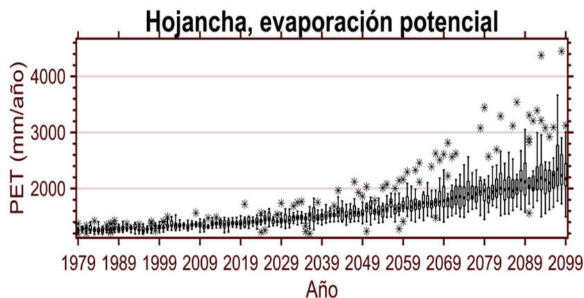
Figura 16. Valores anuales proyectados bajo un escenario pesimista de concentraciones en la evapotranspiración potencial, de 1979 a 2099 promediado para todo el cantón 3
