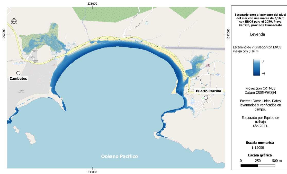
Figura 7. Escenarios de vulnerabilidad ante el aumento del nivel del mar. Marea 3.16 m
