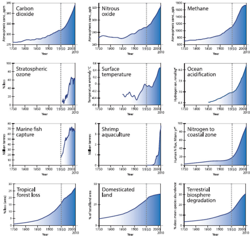
Gráfica No. 3 Consecuencias de la Gran Aceleración en los Ecosistemas Terrestres: dióxido de carbono, óxido de nitrógeno, metano, ozono de la estratósfera, temperatura de superficie, acidificación de los océanos, depredación de peces y crustáceos, nitrógeno en zonas costeras, deforestación, incremento de tierra para agricultura, degradación de la biosfera planetaria. Fuente: http://www.commonhomeofhumanity.org/pdf
